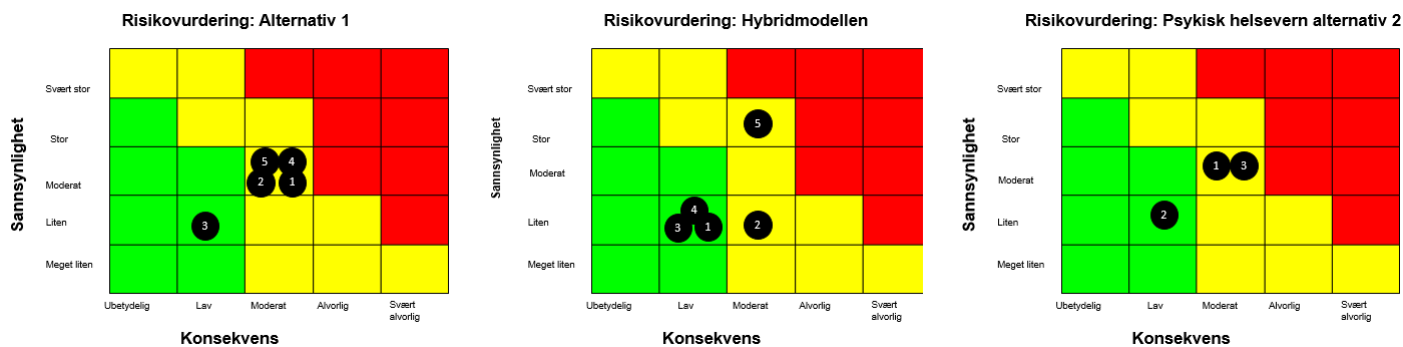
Figur 6. Risikodiagram kapasitet
